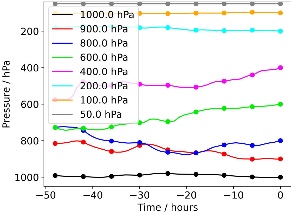
Camborne 20260301_180000
