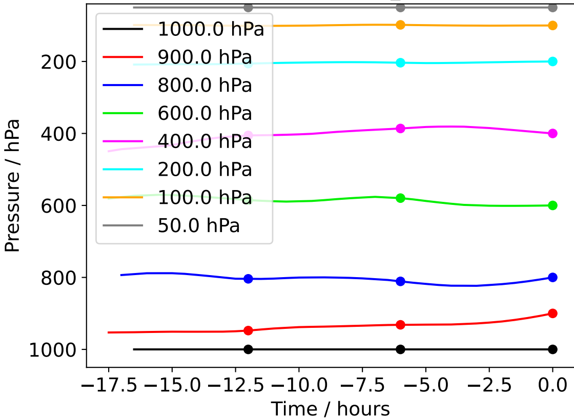
Camborne 20260205_120000
