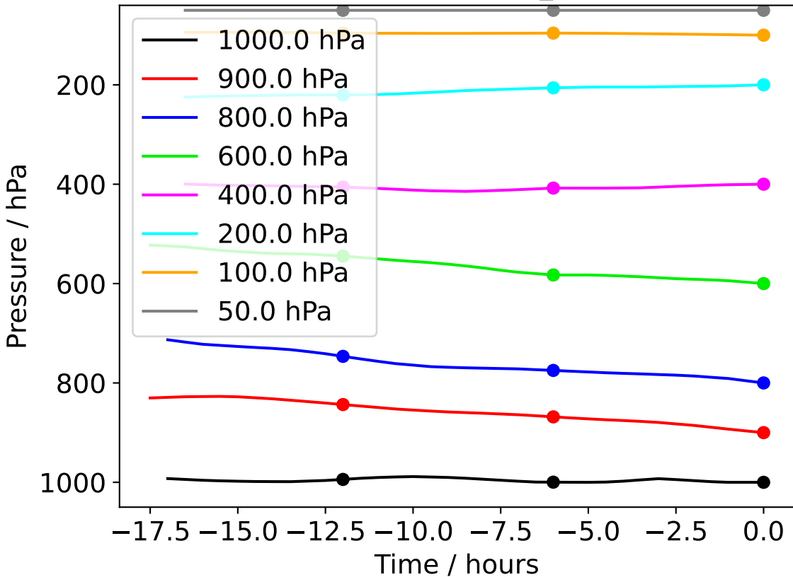
Camborne 20251227_060000
