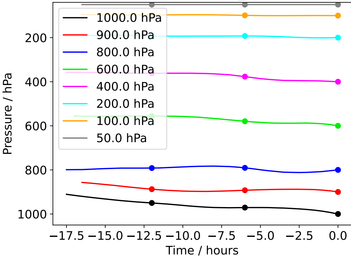
Camborne 20240423_180000
