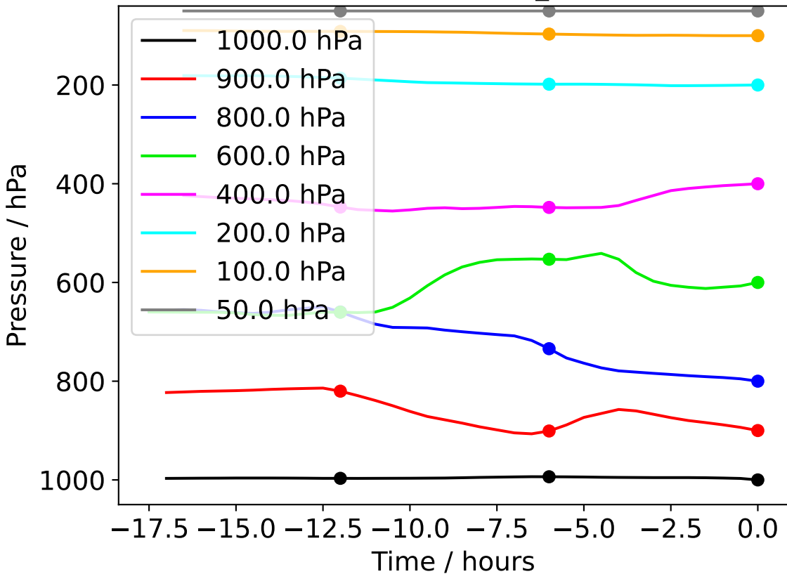
Camborne 20240222_120000
